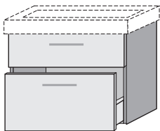
VS203__ 500 x 575 x 425 mm 1 Auszug oben 1 Auszug unten Inneneinteilung unten
