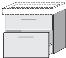
VS202__ 450 x 575 x 390 mm 1 Auszug oben 1 Auszug unten Inneneinteilung unten
