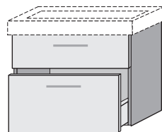
VS204__ 525 x 575 x 450 mm 1 Auszug oben 1 Auszug unten Inneneinteilung unten
