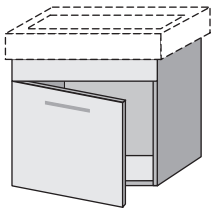
VS200__L 365 x 445 x 300 mm Anschlag links
