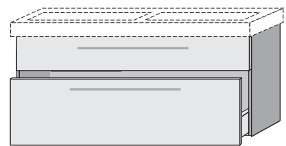
VS207__ 1250 x 575 x 450 mm 1 Auszug oben 1 Auszug unten
