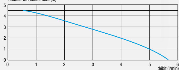
Courbe de débit Sanicondens Eco et Sanicondens Pro hauteur de refoulement (m)
